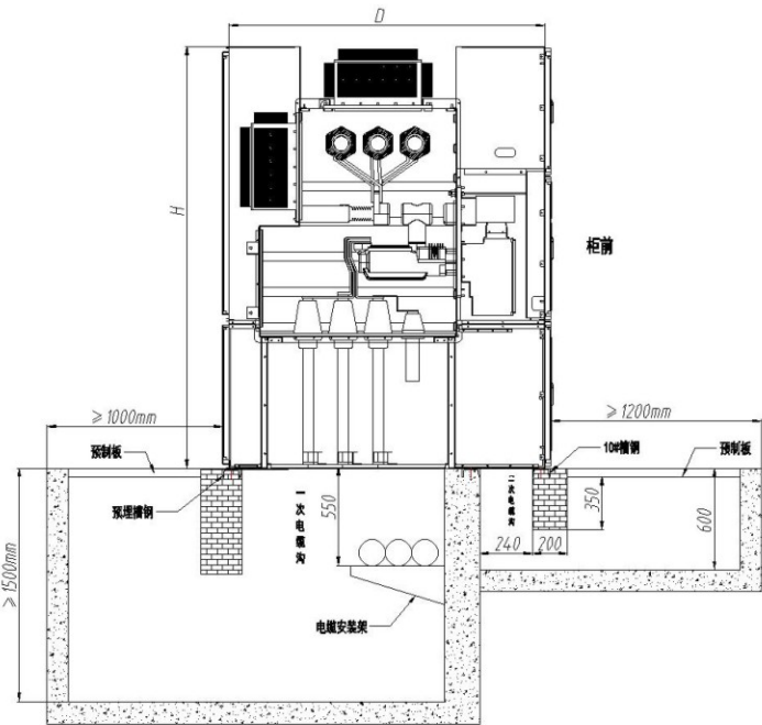
一、地基参考图
