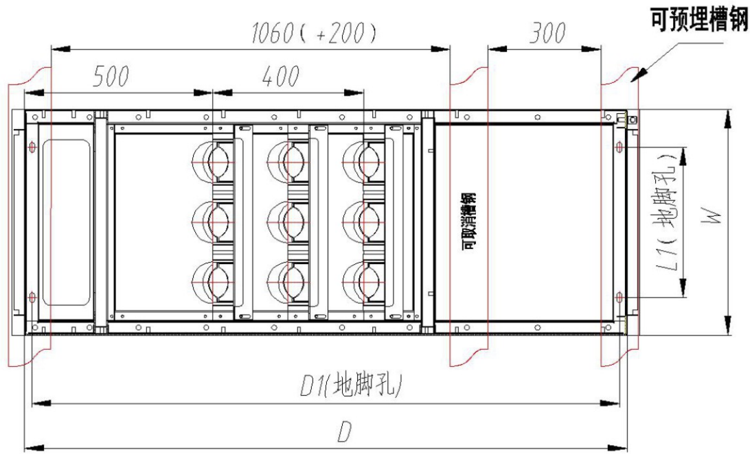
二、基础槽钢示意
