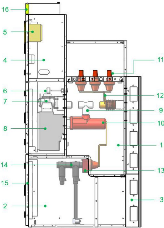
进出线柜（1250A）
